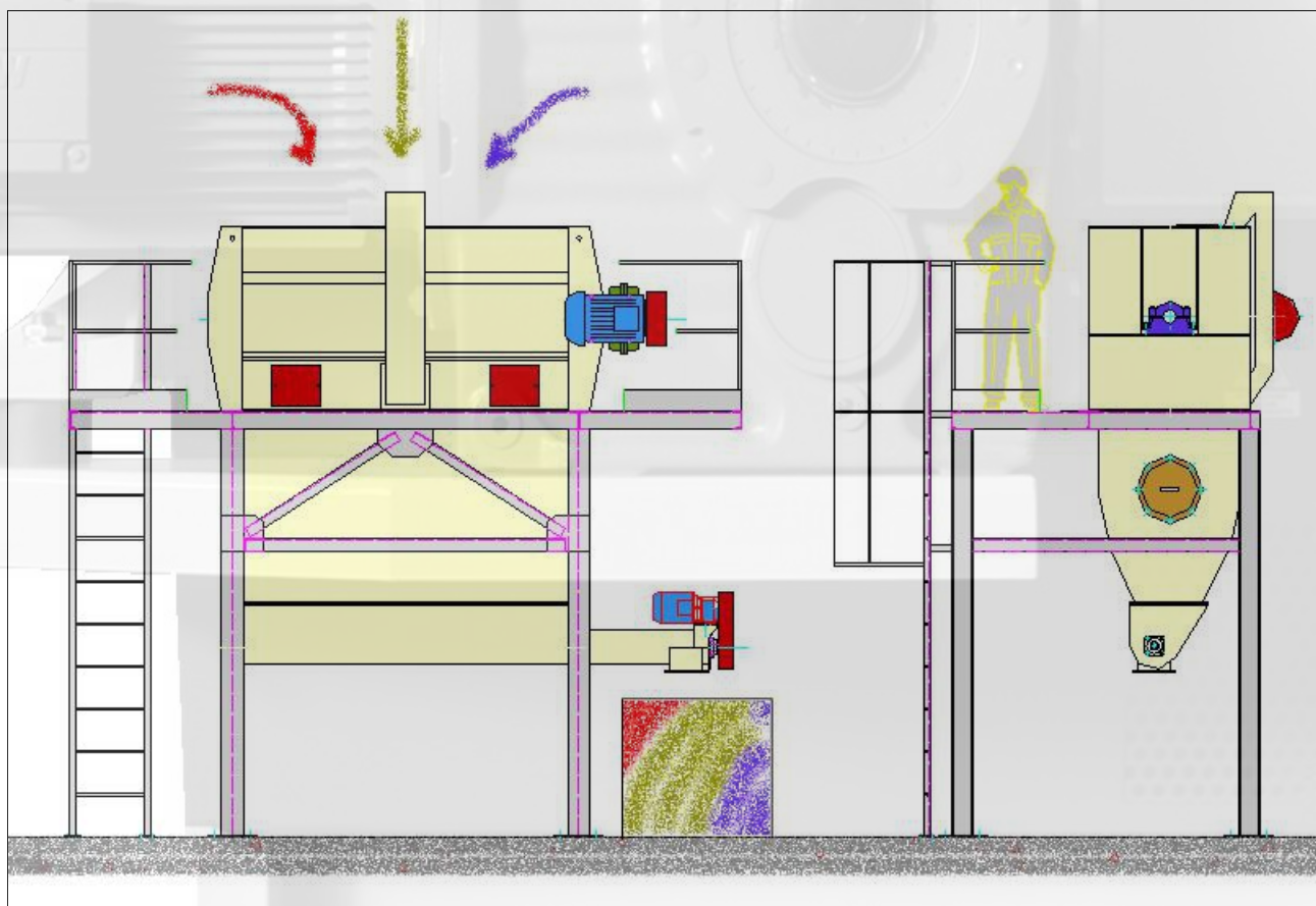
Linea di dosaggio miscelazione e trasporto / Dosing, mixing and conveying line
